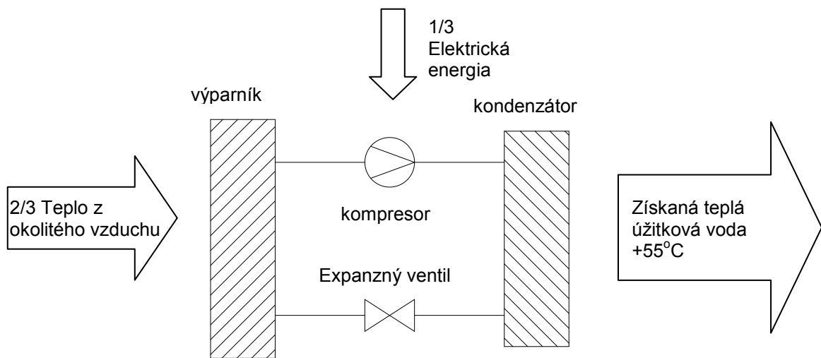
Schéma obehu energie cez agregát tepelného čerpadla
